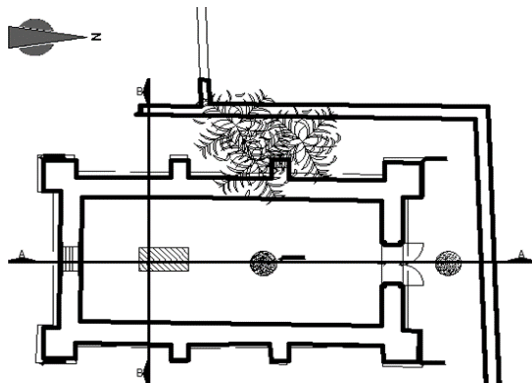
Planta del Antiguo Polvorín
