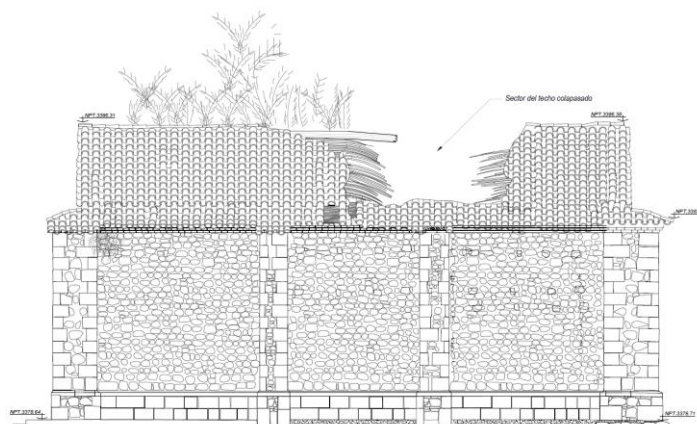
Cerca perimetral y Fachada Principal
