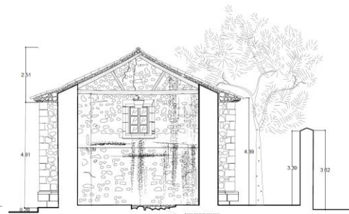
Corte B-B
