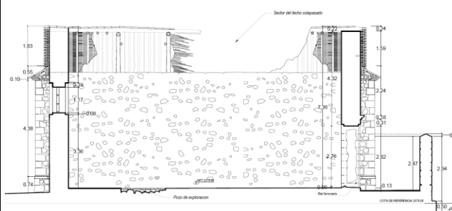
Corte A-A
