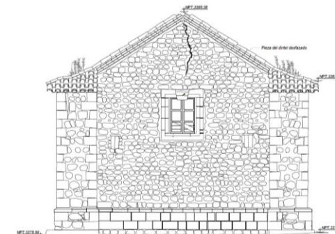
Fachada Posterior
